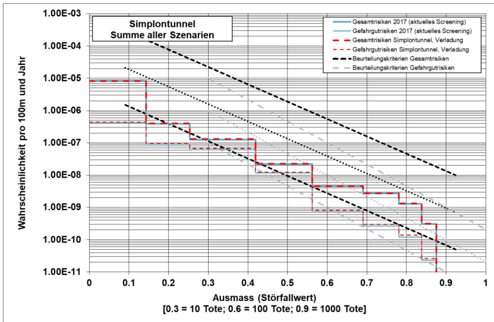
Abbildung 25: W/A-Diagramm der Personenrisiken (Gesamt- und Gefahrgutrisiken) des Simplontunnels bei der Verlagerung auf die Bahn
